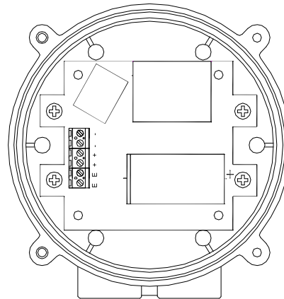
E2xCS112-5EG Beacon Section DC PCB Layout
