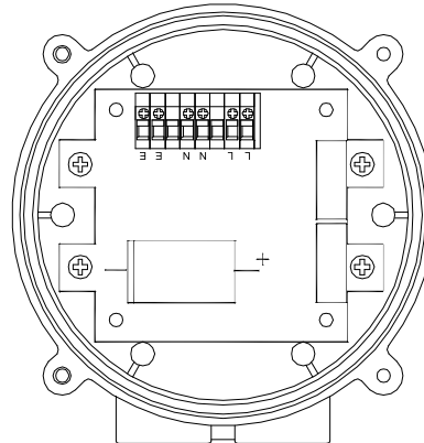
E2xCS112-5EG Beacon Section AC PCB Layout
